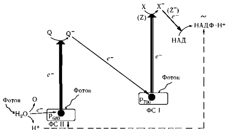
Рис. 228. Z-схема фотосинтеза
