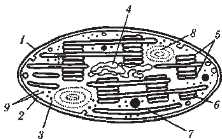
Рис. 221. Строение хлоропласта:
