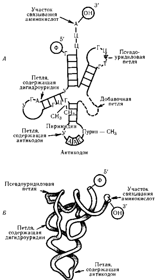
Рис. 206. Структура тРНК:
